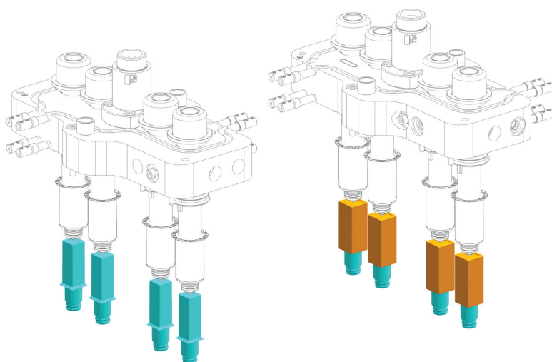
Application de bouteilles à plusieurs matériaux de 4+4 cavités
