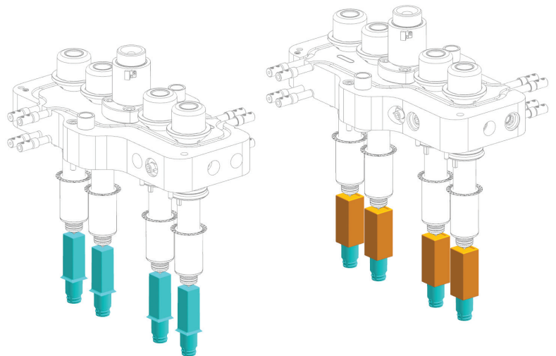
Aplicación de botella multimaterial de 4+4 cavidades
