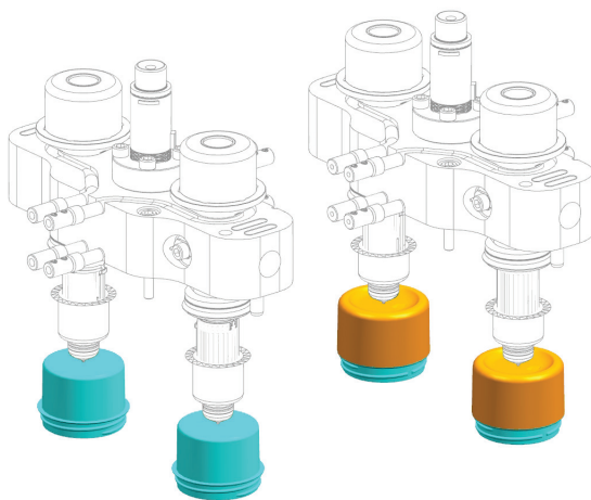
Aplicación de tapa multimaterial de 2+2 cavidades
